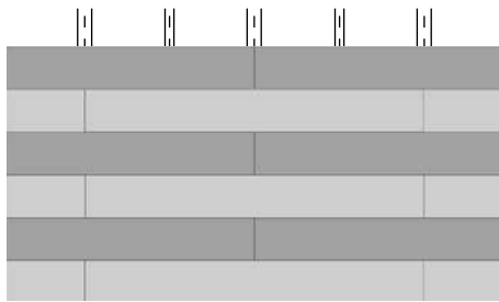
Halber Verband
